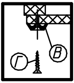
Крепление задней стенки (комплект №10)
