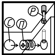
Крепление стяжки эксцентри- ковой (комплект №4,5)
