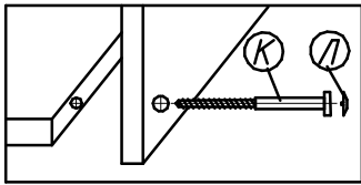
Крепление винта саморезного (комплект №19)
